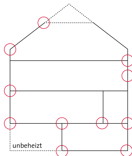
▲ Wärmebrücken
