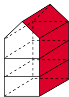
▲ Gebäude freistehend > 350m 2 0,5 \text{ W}/(\text{m}^2 \cdot \text{K})
