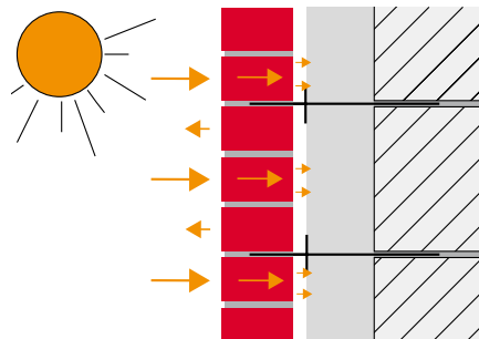
▲ Sommerlicher Wärmeschutz
